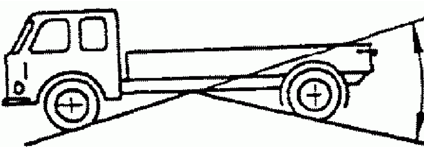
Рис. 3. Продольный угол проходимости
